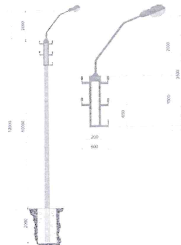
Опора из ж/б
